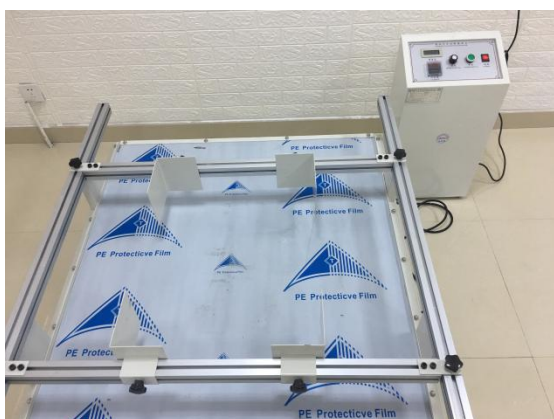
模拟汽车运输震动台
